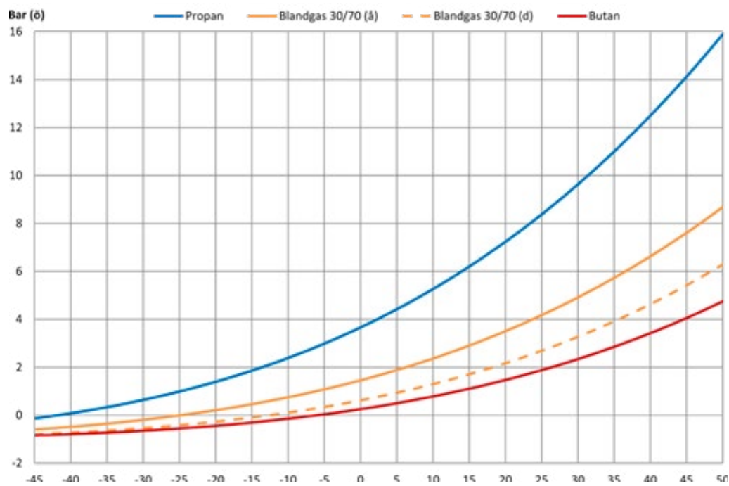
Figur 3.5 Ångtrycksdiagram
